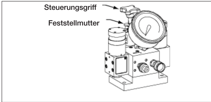
Abb. 12, Überdruckventil
