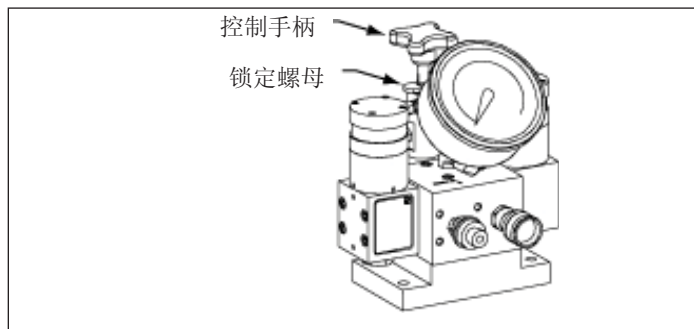
图12- 泄压阀
