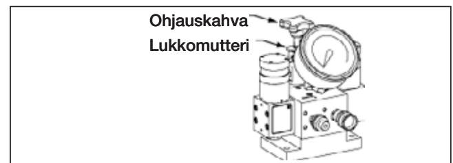
Kuva 12, Varoventtiili
